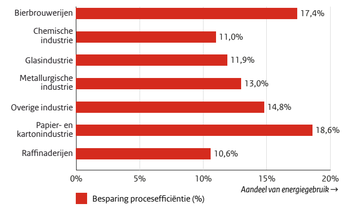
Figuur 2.7 – Besparing door procesefficiëntie MEE-sectoren in PJP en % . Referentiejaar 2009, t.o.v. eigen energiegebruik sectoren
