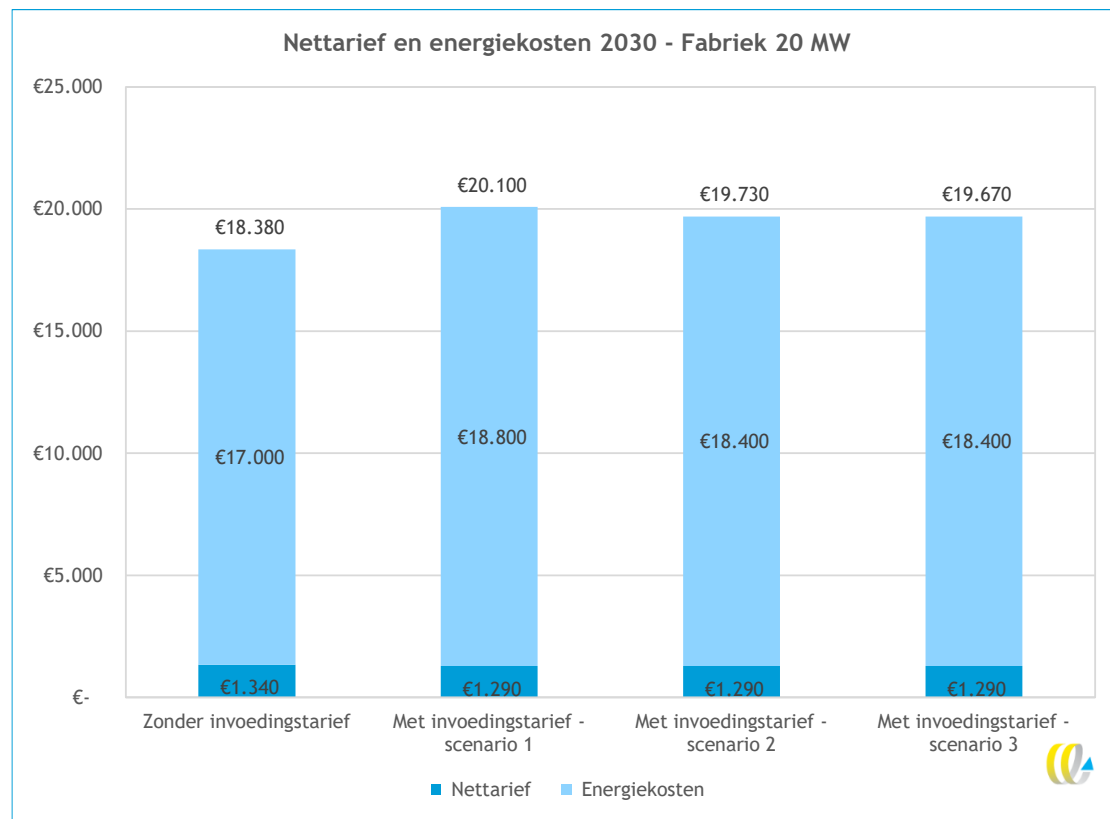
Figuur 16 - Nettarief en energiekosten van de casus 'Fabriek 20 MW'. Afgerond op tiental euro's
